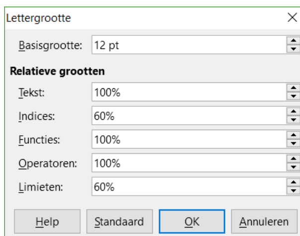
Afbeelding 7: Dialoogvenster Lettergrootte
