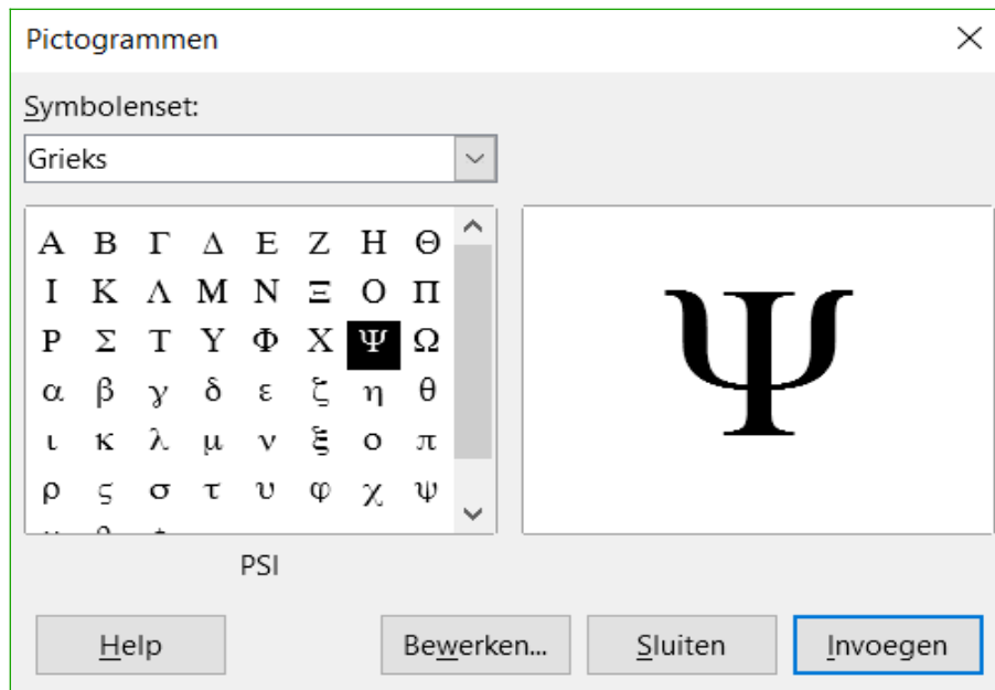
Afbeelding 4: Dialoogvenster Pictogrammen
